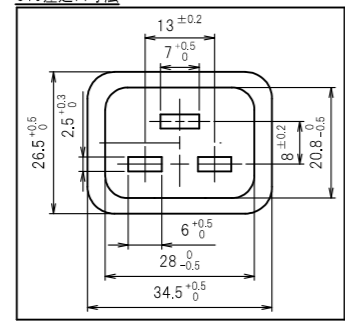
C19差込口寸法
