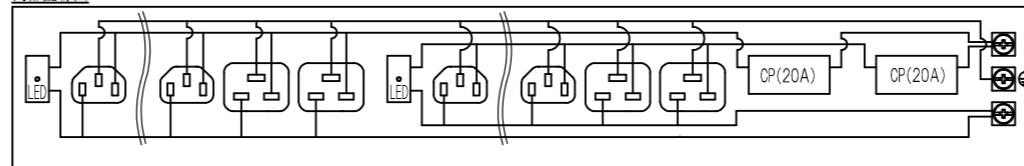
内部配線図
