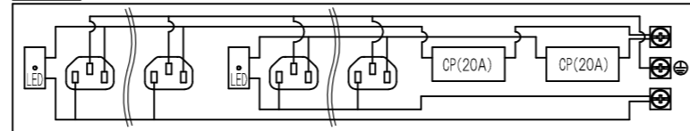
内部配線図
