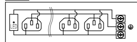
内部配線図
