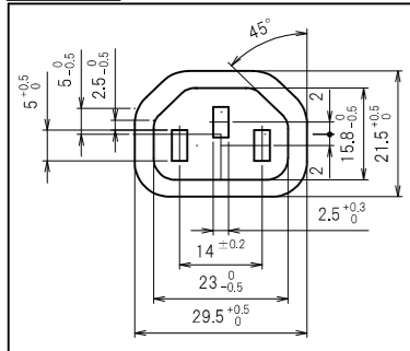
C13差込口寸法
