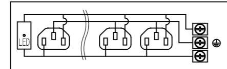
内部配線図
