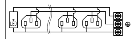
内部配線図
