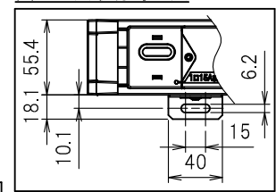
圧着端子カシメ位置寸法
