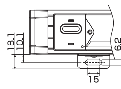
本体取付穴寸法
