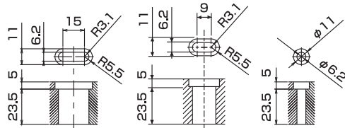
本体取付穴寸法
